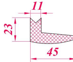
Прокладка уплотнительная АВТМ - 1600
