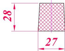
Профиль 27/24 × 28
