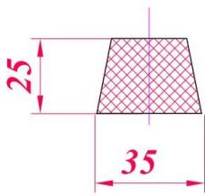
Профиль 35/25 × 25
