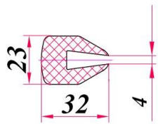
Накладка 5276.02.00.004
