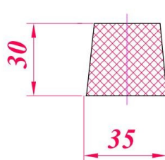
Профиль 35/28 × 30
