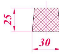
Профиль 30/25 × 25
