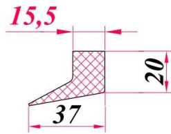
Уплотнитель автоклава 37 × 20 × 15,5
