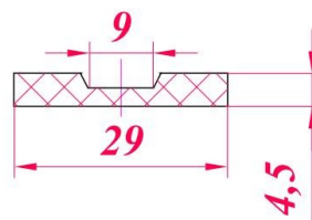
Профиль - прокладка ПРК - 2 ( 6208 - 61 )
