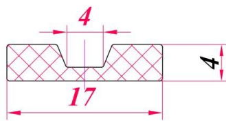
Профиль - прокладка ПРК - 1 ( 5208 - 61 )
