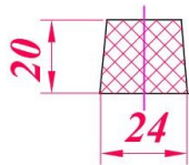
Профиль 24/20 × 20
