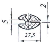
Уплотнитель НТ-10
