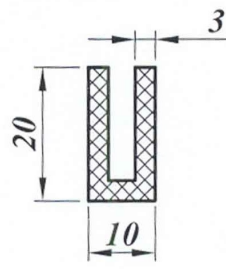
Профиль 20 × 10 × 3
