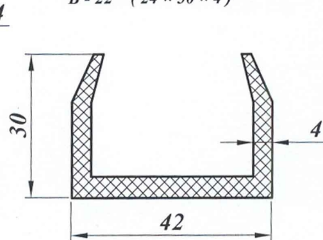
Окантовка стеклопакета В-34 (30 × 42 × 4) (Д4101 - 761)
