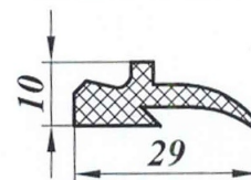
Уплотнитель НТ-8
