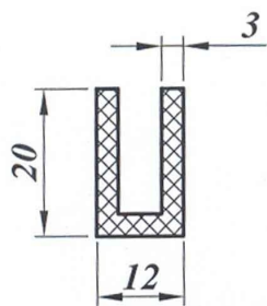
Профиль 20 × 12 × 3
