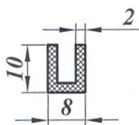
Профиль 10 × 8 × 2
