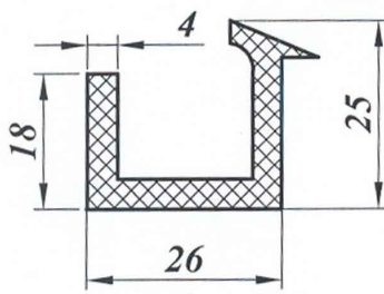
Окантовка стеклопакета В-18 (18 × 26 × 4)
