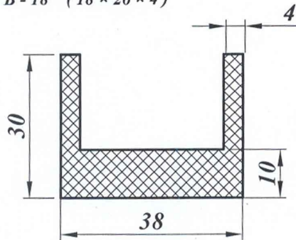
Окантовка стеклопакета В-30 (30 × 38 × 4)
