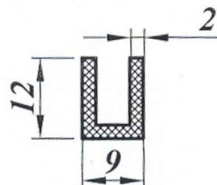
Профиль 12 × 9 × 2
