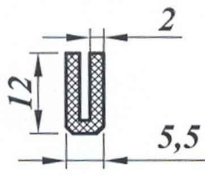
Профиль 12 × 5,5 × 2
