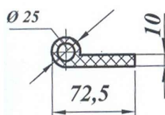
Уплотнение гидрозатвора ГС
