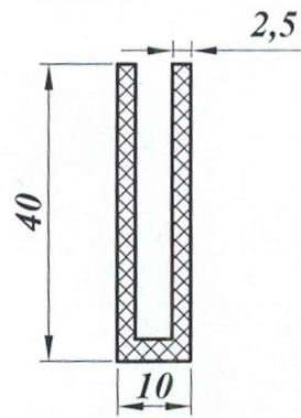
Профиль 40 × 10 × 2,5
