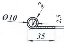
Кант уплотнительный
