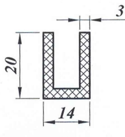
Профиль 20 × 14 × 3
