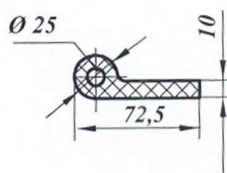
Уплотнение 3ЗБВ-06 ГС
