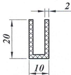
Профиль 20 × 10 × 2
