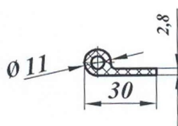
Уплотнитель АУЗС 2М-131-129
