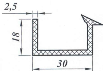
Окантовка стеклопакета В-25 (18 × 30 × 2,5)
