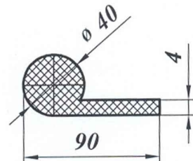
Профиль опорный
