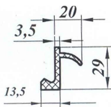
Профиль Р2-125 (Р-14, Р-14-000)
