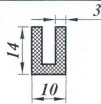
Профиль 14 × 10 × 3
