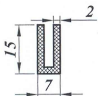
Профиль 15 × 7 × 2
