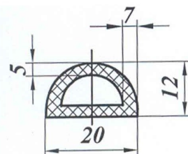
Профиль опорный
