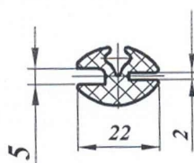
Уплотнитель НТ-9
