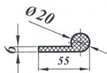
Уплотнение ГС 40.03.003-01
