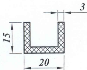
Окантовка стеклопакета В-14 (15 × 20 × 3)
