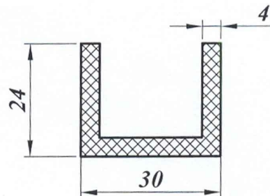
Окантовка стеклопакета В-22 (24 × 30 × 4)
