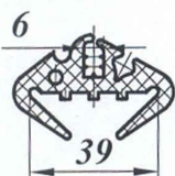
Профиль ПР-015 (682-5403398)
