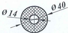
Упор Т2-14-264
