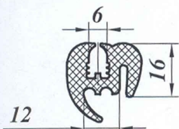
Уплотнитель 01-013-011 (Н-418)
