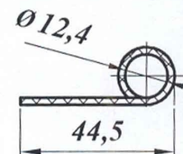
Уплотнитель ПР-057 (НТ-18)
