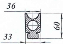
Уплотнение 608.11.08.011
