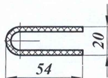
Профиль ПР-042
