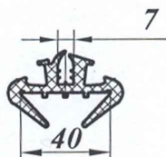
Профиль ПР-186
