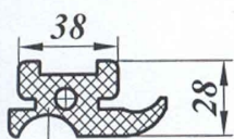
Уплотнитель 605.11.68.228
