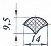
Уплотнитель ПР-187
