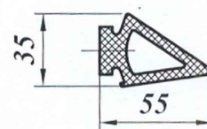
Уплотнитель ПР-249
