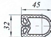
Уплотнение Н-771
