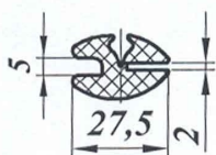
Уплотнитель НТ-10
