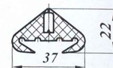
Профиль ПР-38
