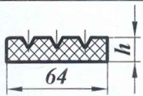
Профиль 605.09.00.028 h=15 Профиль 605.09.00.028-1 h=10 Профиль 605.09.00.028-2 h=13,5
