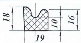
Уплотнитель ПР-072 (пористый)
