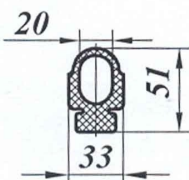
Уплотнение 608.11.08.010
