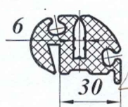
Профиль УКПР 008-66 (71-605)
