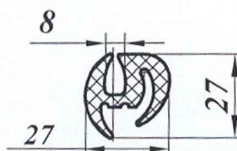
Уплотнитель 01.015.022
