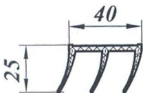
Уплотнитель двери 3-х лепестковый
