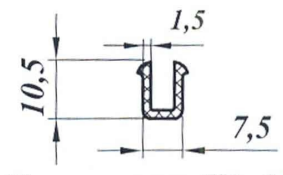
Уплотнитель ПР-030
