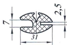
Уплотнитель ПР-77 (500-5206018-27), (ПР-22, СТП-37)
