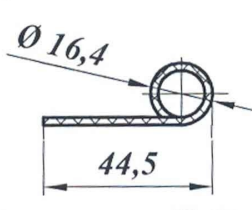
Уплотнитель Н-18 (ПР-058, ПР-057)
