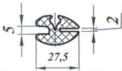
Уплотнитель НТ-10 (ПР-008)
