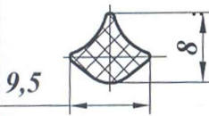
Замок уплотнитель РСМ-10.04.44.002
