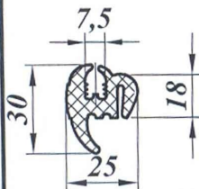
Уплотнитель ПР-099 (250-5206054-10)
