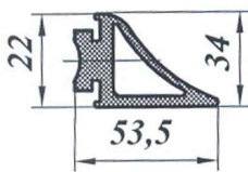
Уплотнитель ПР-248 (5256-6107052)
