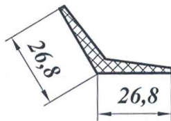
Уплотнитель двери 677-6107140-Б
