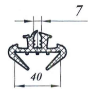
Профиль ПР-186
