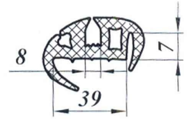
Уплотнитель ПР-144-10
