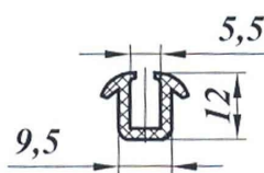
Уплотнитель ПР-032
