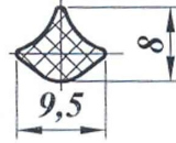
Уплотнитель НТ-8 (ПР-028)
