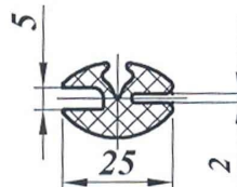
Уплотнитель стекол РСМ 10Б.01.44.002
