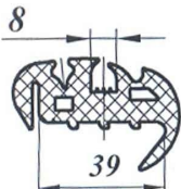
Уплотнитель ПР-157
