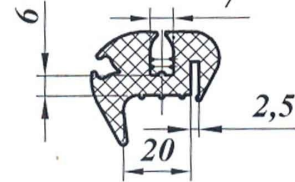
Уплотнитель ПР-019
