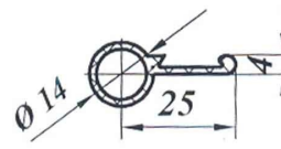
Профиль ПР-14
