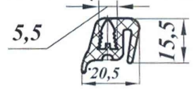
Уплотнитель 038НП 101-62
