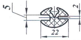
Уплотнитель НТ-9 (ПР-005)
