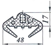
Уплотнитель ПР-015
