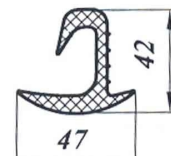
Уплотнитель двери рефрижираторов.
