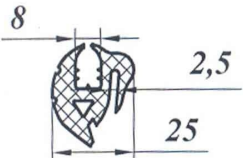
Профиль 038НТ-102-90
