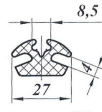
Уплотнитель ПР-260 (377-5206055-A)
